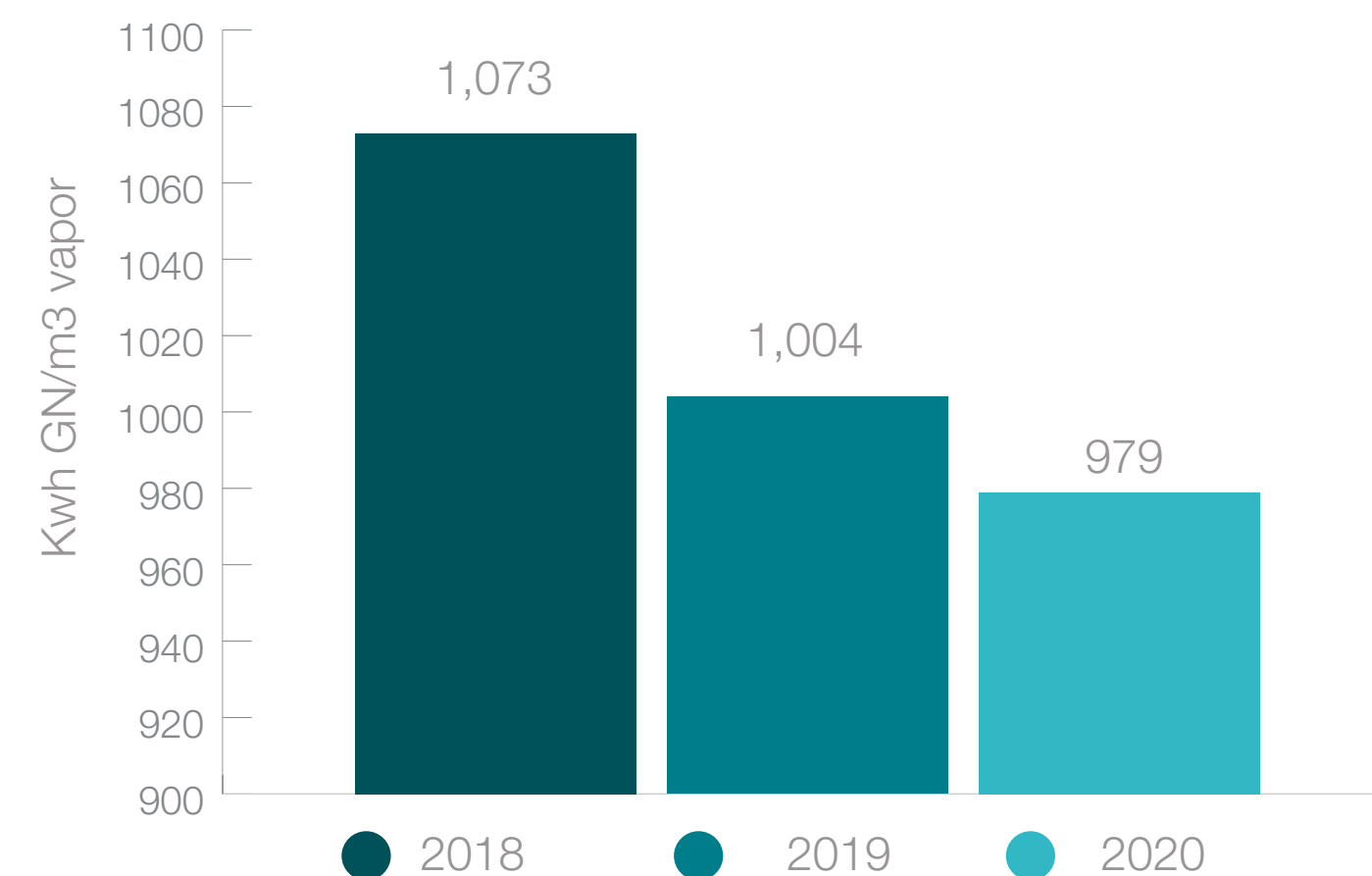
Calderas de Vapor Aqua (Kwh Gas Natural/ m3 vapor)
